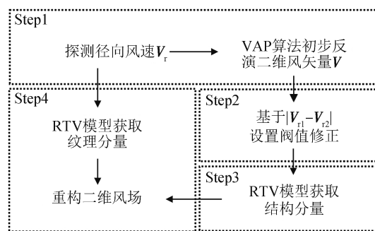
图2 算法流程图
